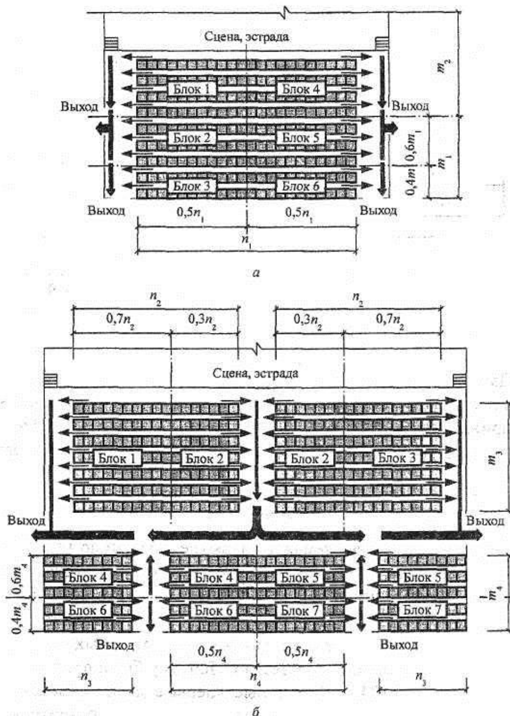
Рисунок Ж. 1. - Маршрутизация движения людских потоков при эвакуации из зрительных залов а – с боковыми (продольными) проходами; б - с поперечным проходом
