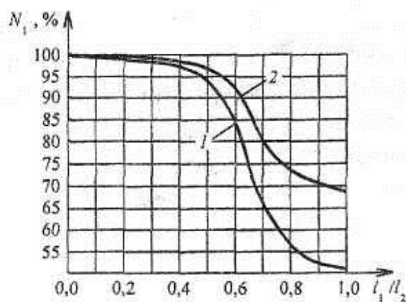
Рисунок Ж. 2. - Распределение числа зрителей между выходами
